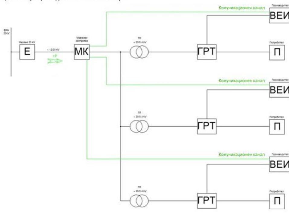
2). Схема при присъединяване на Обекта на СРН:
