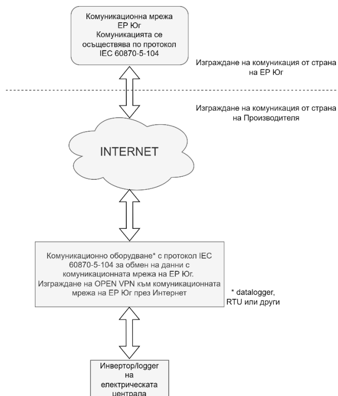
Фигура 4: Изграждане на комуникационна връзка обект за производство или съхранение на електрическа енергия – комуникационна мрежа ЕР Юг
