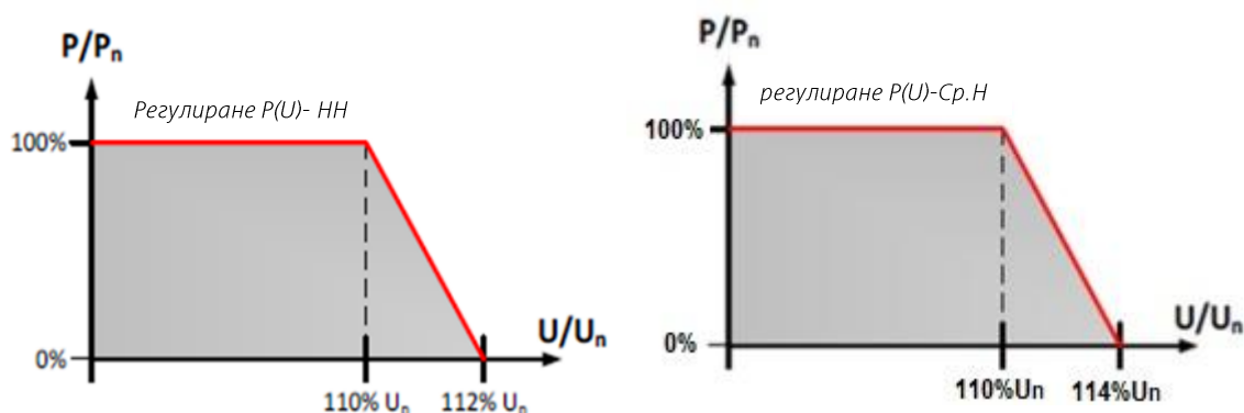
Фигура 3:Настройки за регулиране P(U)
