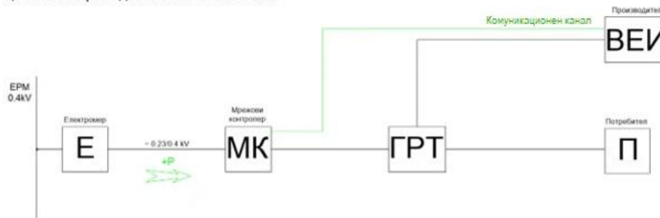
1). Схема на присъединяване на Обекта на НН:
