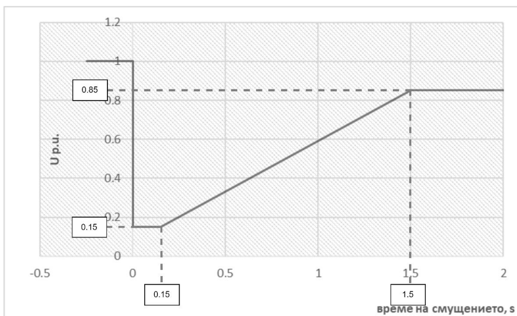
Фигура 1: FRT-профил на несинхронен генератор, присъединен в мрежа МН
